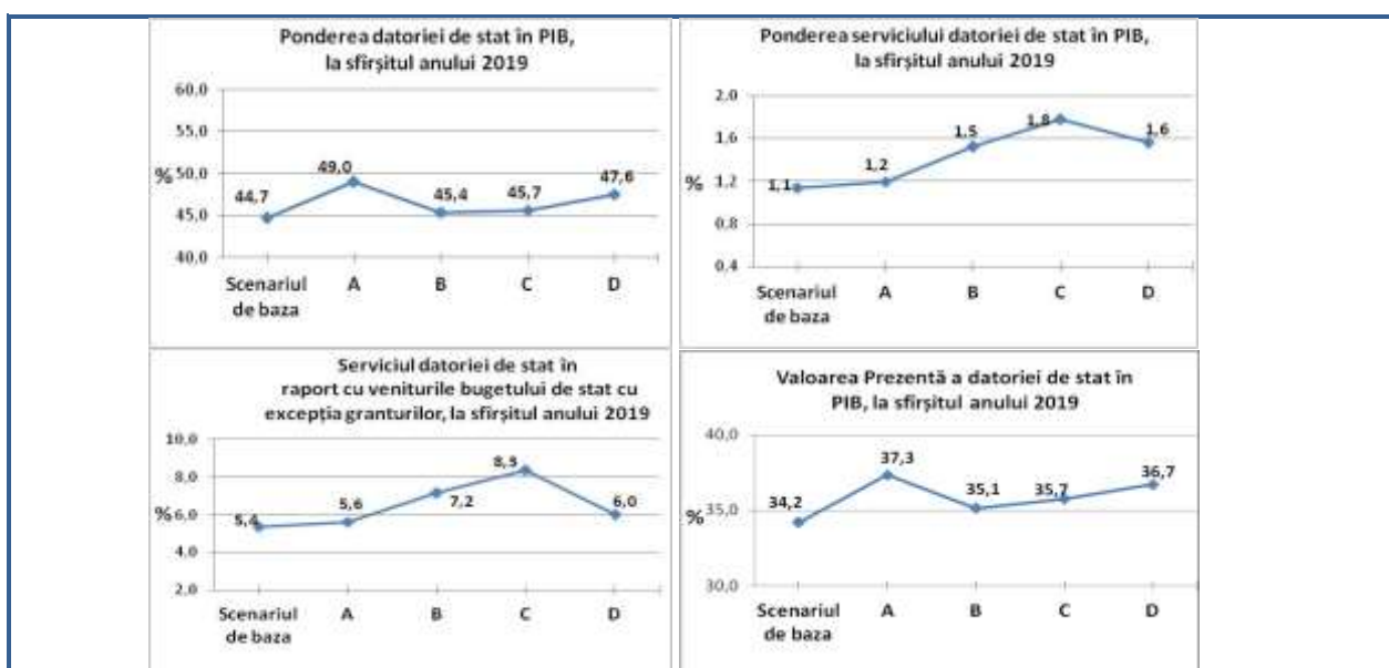
Fig. 2. Evoluția indicatorilor datoriei de stat ca rezultat al aplicării S1 și sub influența șocurilor privind evoluția indicatorilor de piață, conform situației de la sfîrșitul anului 2019
