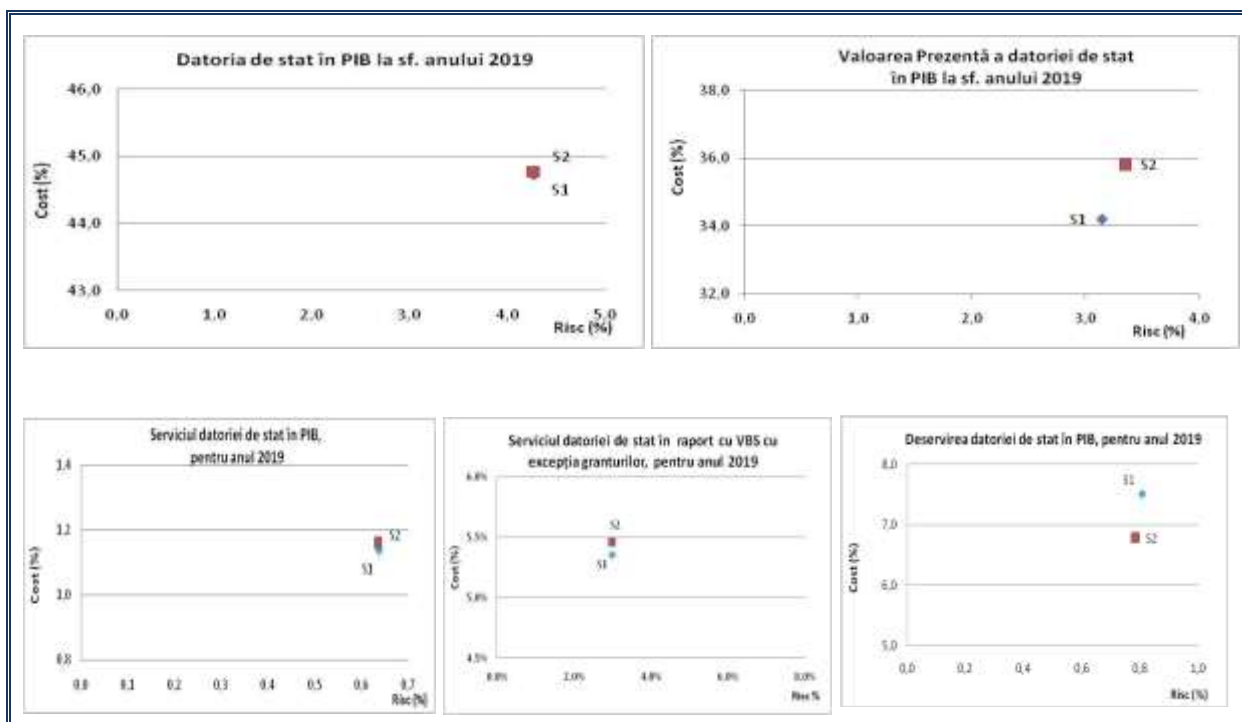
Fig.1. Evoluția indicatorilor datoriei de stat ca rezultat al aplicării strategiilor de finanțare S1 și S2
