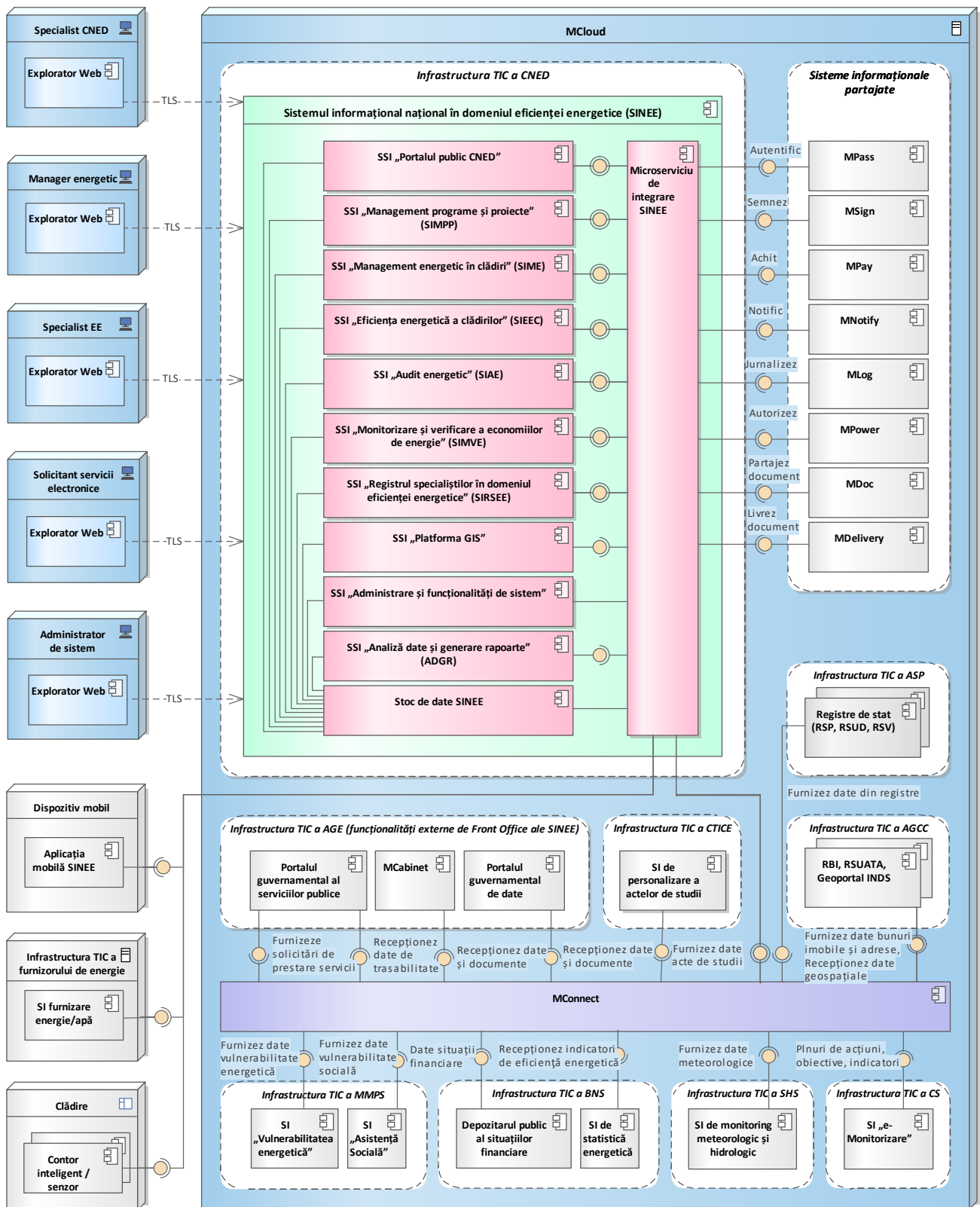
Figura nr. 14. Arhitectura SINEE.
