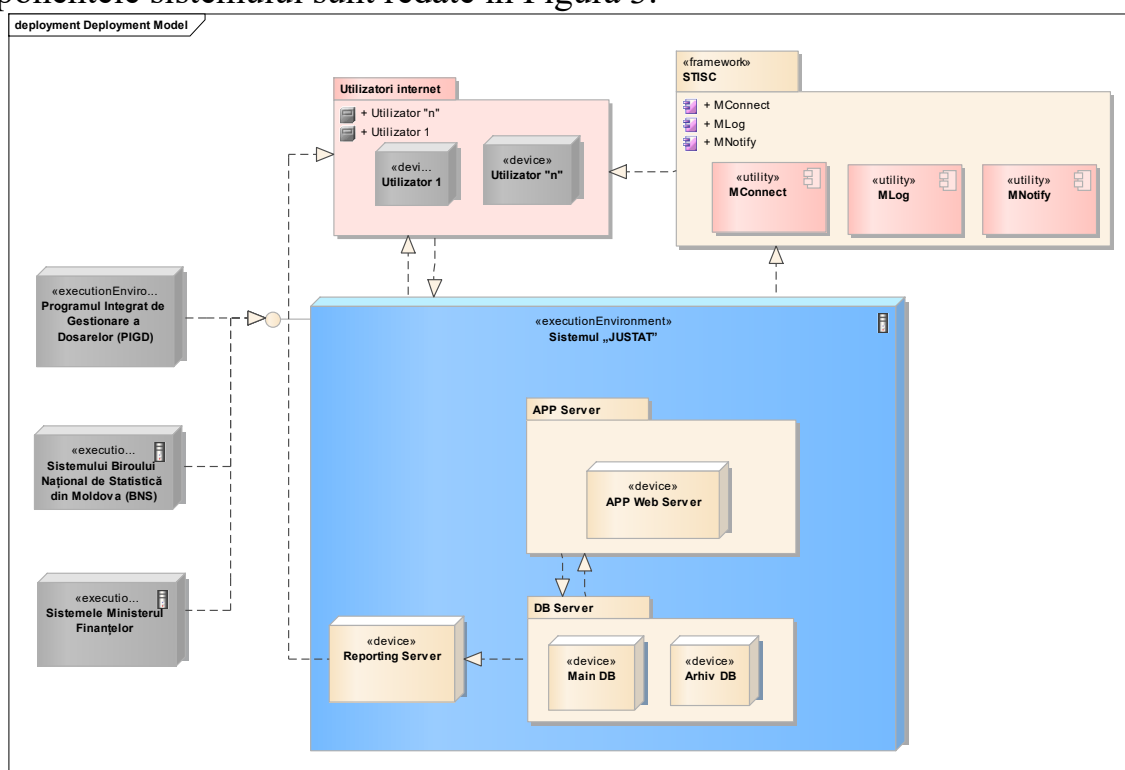
Figura 3 – Arhitectura și componentele SI JUSTAT
